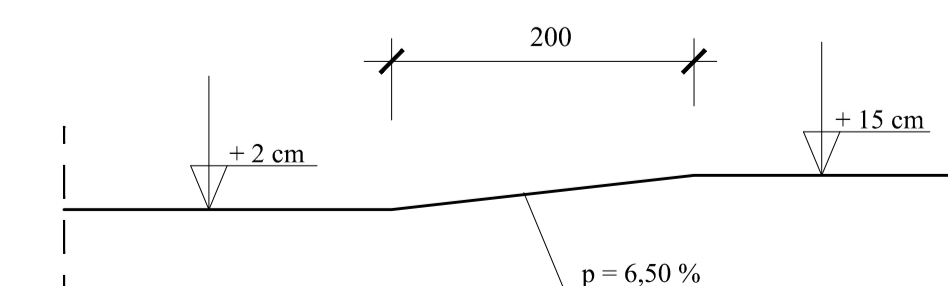
SEZIONE X-X 1:50
