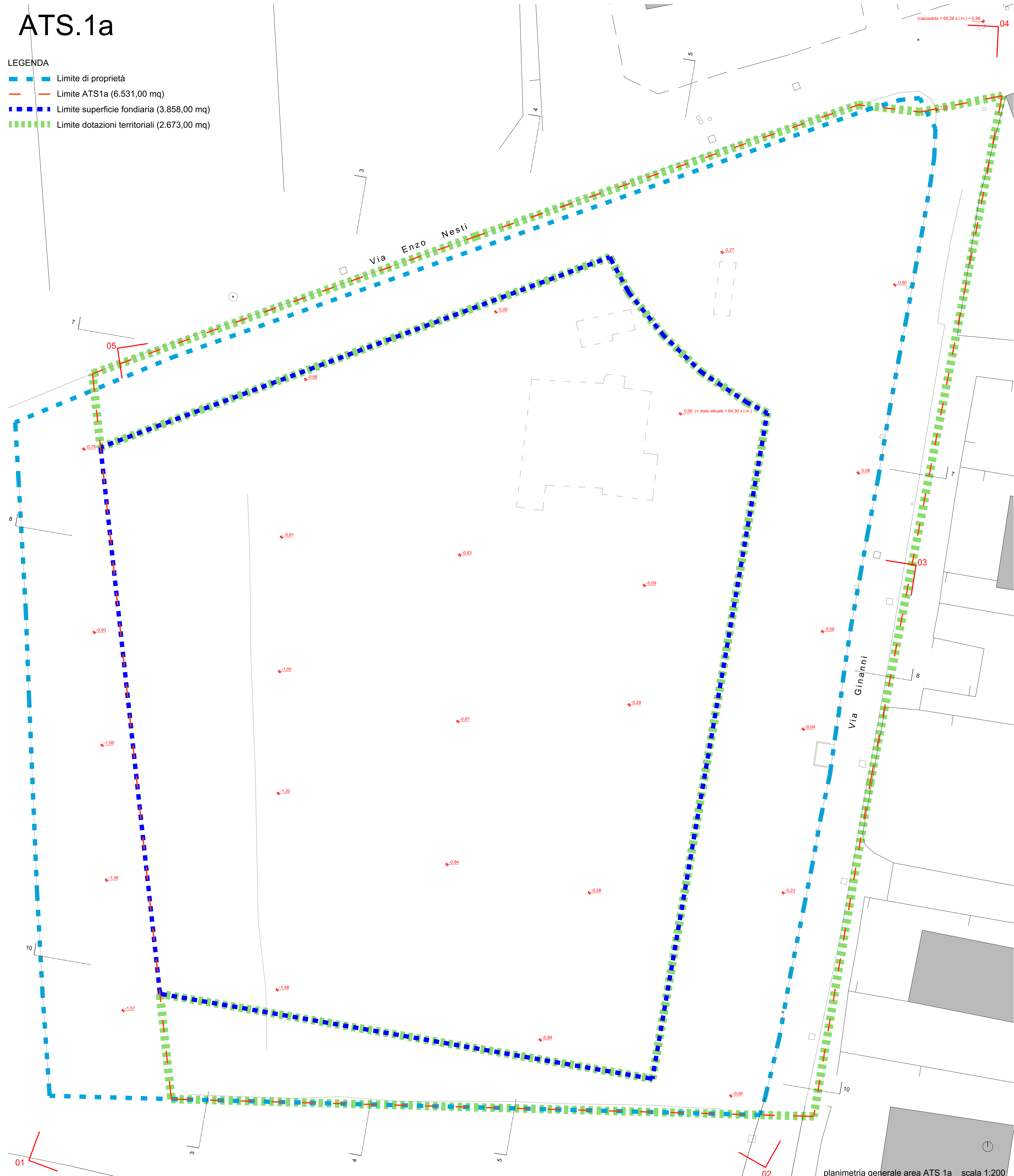
planimetria generale area ATS 1a scala 1:200
